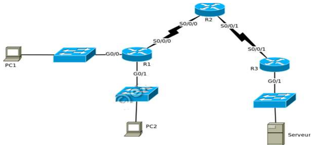
ACL IPv6
